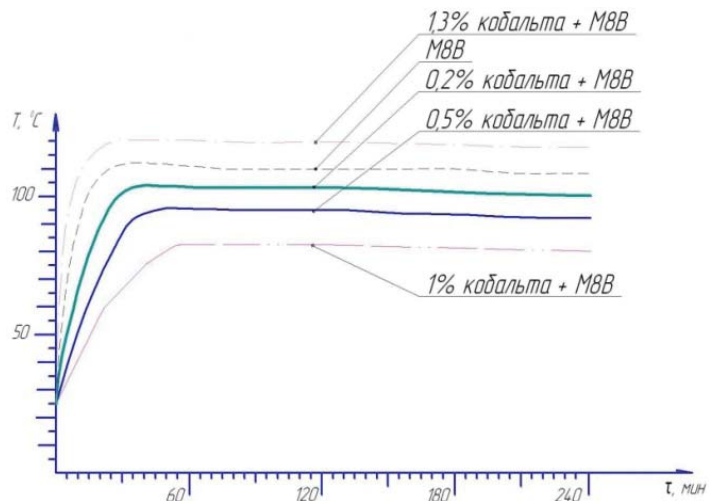
Рис. 2. Изменение температуры ( T ) в зоне контакта от времени испытаний ( t ) при различном содержании нанокобальта в масле М8В: нагрузка N = 900 Н, скорость скольжения v = 1,5 м/с
