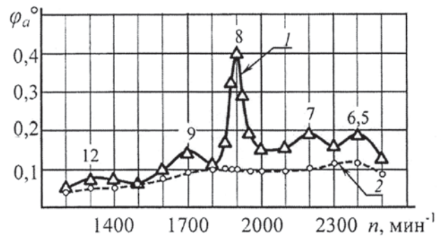
Рис. 3. Амплитуда угла закрутки носка коленчатого вала при работе дизеля по ВСХ: 1 и 2 – соответственно без демпфера и с демпфером крутильных колебаний; 6,5; 7; 8; 9; 12 – номера резонирующих моторных гармоник
