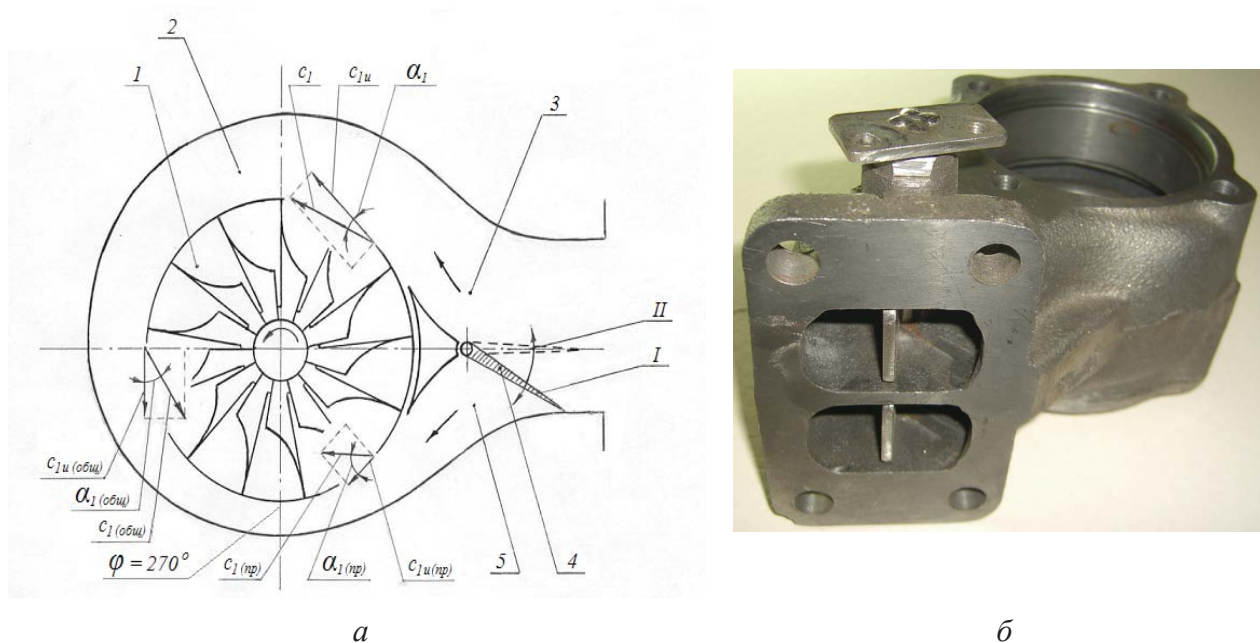
Рис. 1. Схема способа регулирования (а) и корпус турбины (б)
