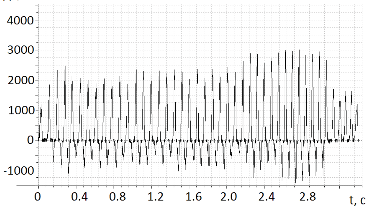
Рис. 1. Фрагмент осциллограмм изменения моментов на торсионном валу (в процессе пуска-остановки двигателя)
