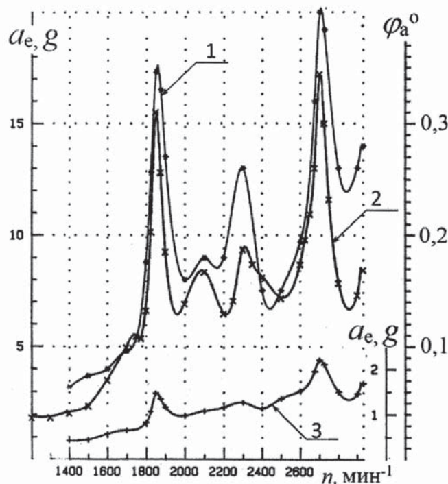
Рис. 10. Связь угла закрутки носка коленчатого вала и вибраций на стяжном болте:
