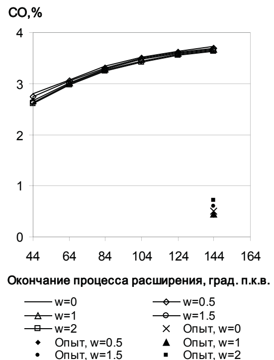
Рис. 1. Теоретические и экспериментальные данные содержания оксида углерода в ОГ дизеля при впрыскивании воды на режиме максимального крутящего момента
