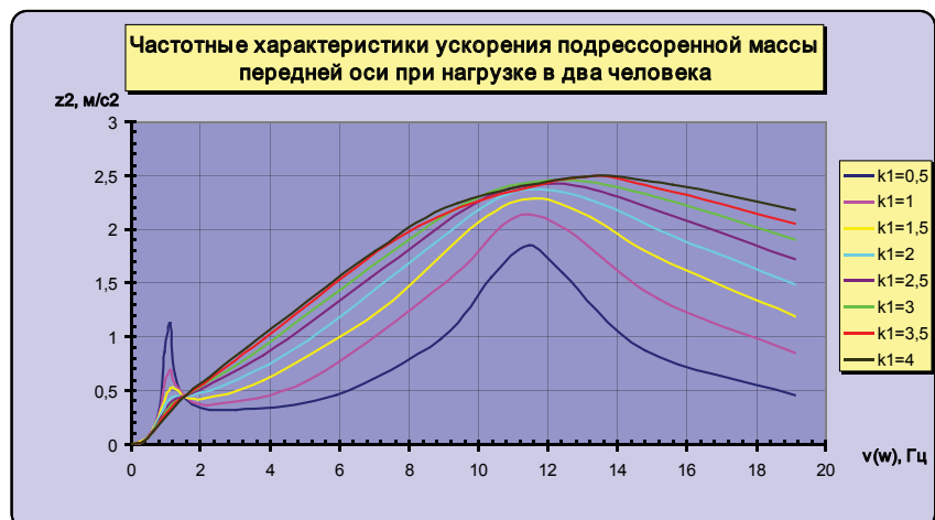
Рис. 1. Пример характеристики ускорения поддресоренной массы
