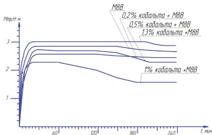
Рис. 1. Изменение момента трения ( M_{тр} ) в зоне контакта от времени испытаний ( t ) при различном содержании нанокобальта в масле М8В: нагрузка N = 900 Н, скорость скольжения v = 1,5 м/с
